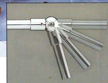
Barre raidisseur 3 volumes à angle réglable Reinforcement bar for 3 panels with adjustable angle
